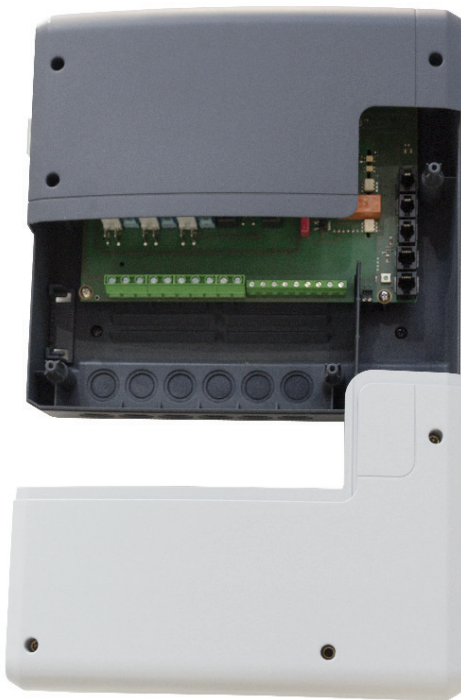
Leistungsteil, Unterteil der Frontabdeckung geöffnet
